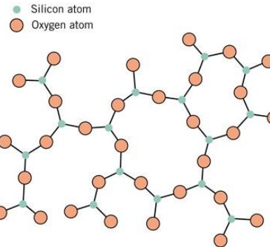
noncrystalline SiO 2
